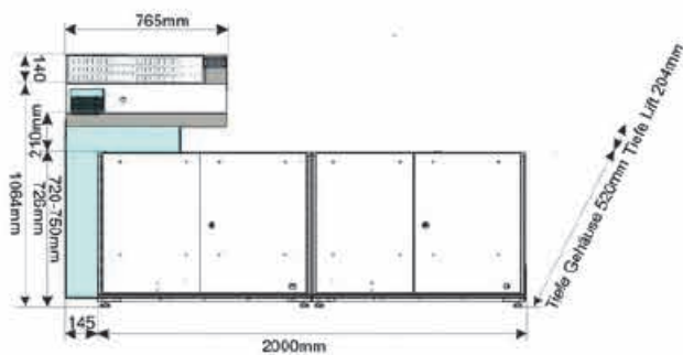
SMT Untertisch-Version 84
